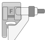
暗线缝压脚 (F) 暗线缝压脚用于在衣服和家饰中缝制暗线。正面有一个带延长的可调节导杆，用于在缝制过程中引导折叠卷边。
